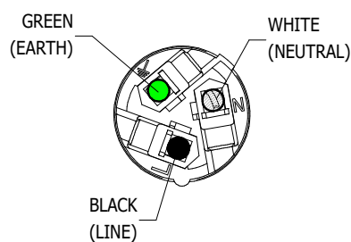
UL WIRING
