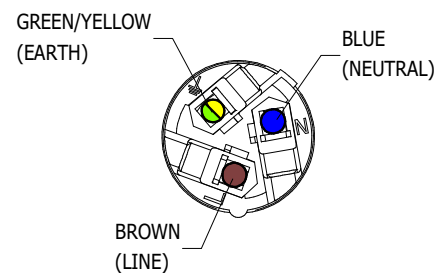
VDE WIRING
