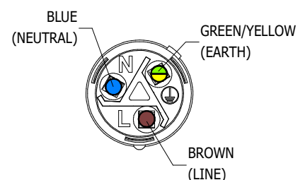
VDE WIRING
