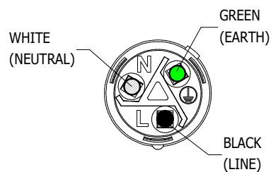
UL WIRING
